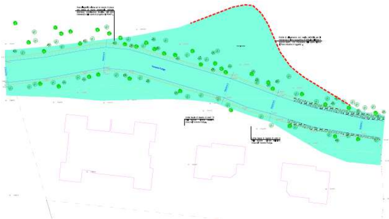
Dettaglio estratto dalla Tav. n. 2: Aree Allagabili TR=100 – Torrente Pudiga
