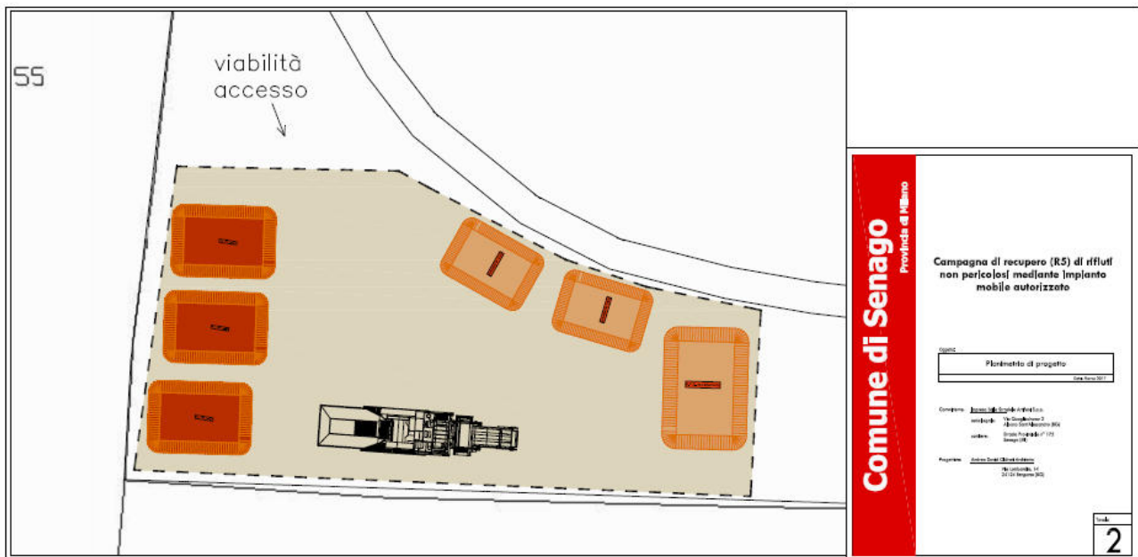
Tavola 2 - Planimetria di progetto
